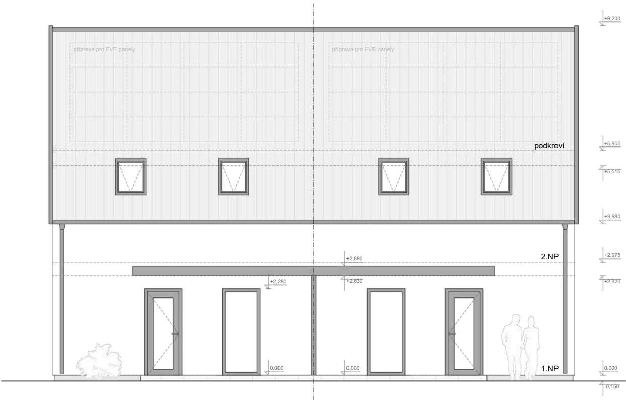
POHLED.Z ULICE
